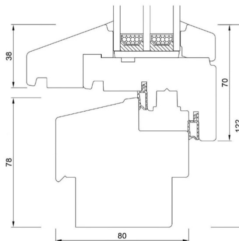
Systemschnitt unten
