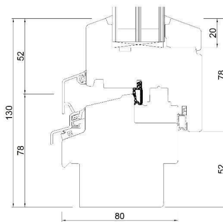
Systemschnitt unten
