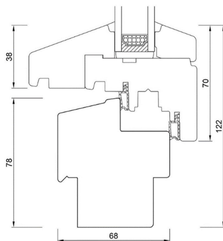
Systemschnitt unten
